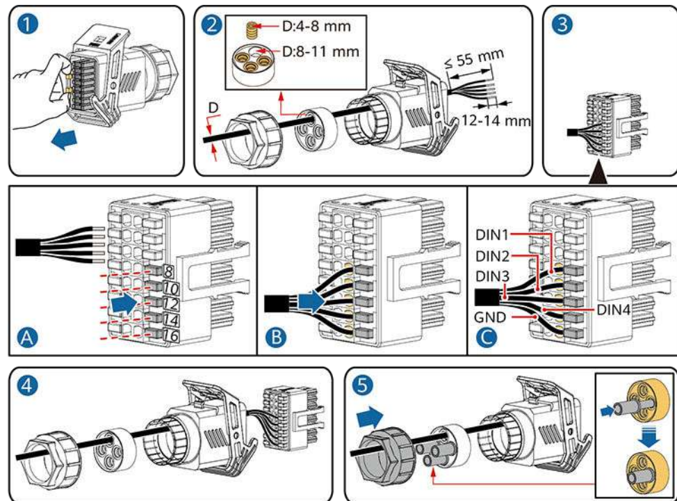
Figura 5-34 Instalación del cable
