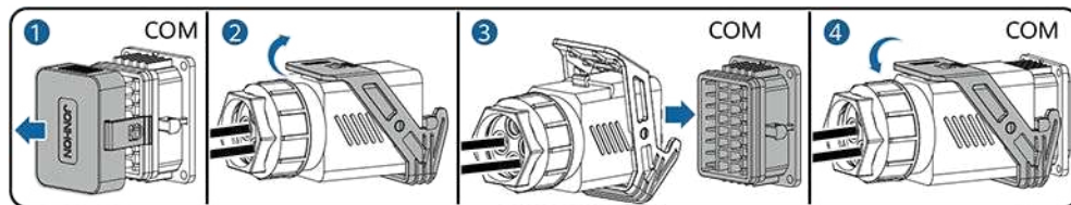
Figura 5-32 Fijación del conector del cable de señal
