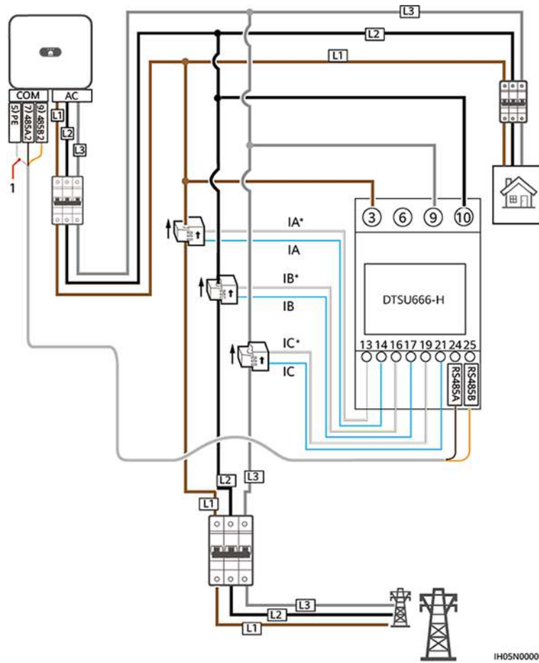
Figura 5-23 Conexión trifásica y trifilar (conexión en red del Smart Dongle)
