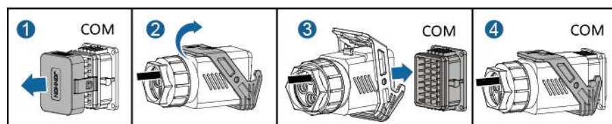
Figura 5-35 Cómo ajustar el conector del cable de señal
