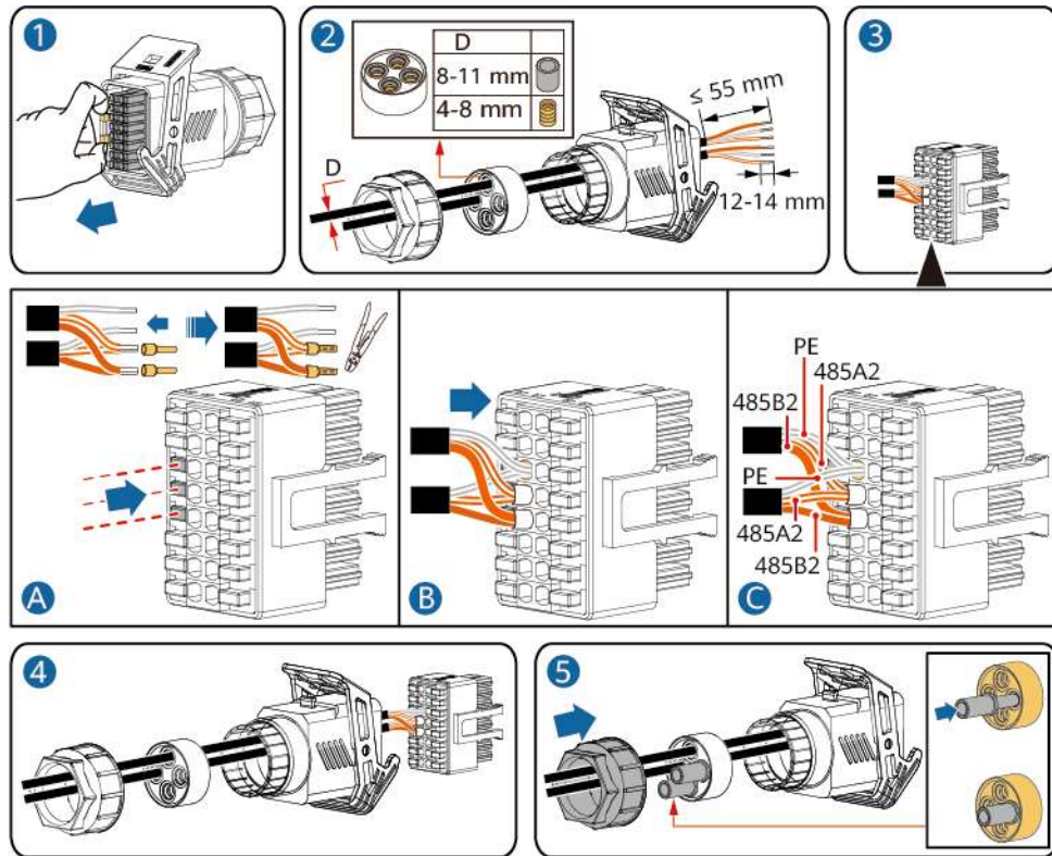
Figura 5-31 Instalación del cable
