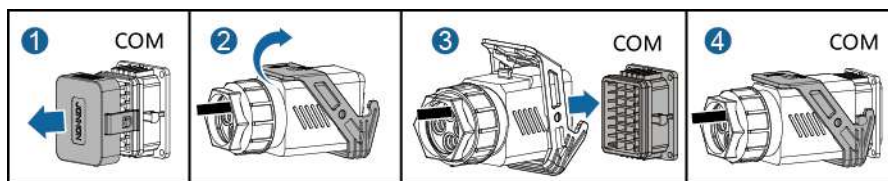
Figura 5-37 Fijación del conector del cable de señal
