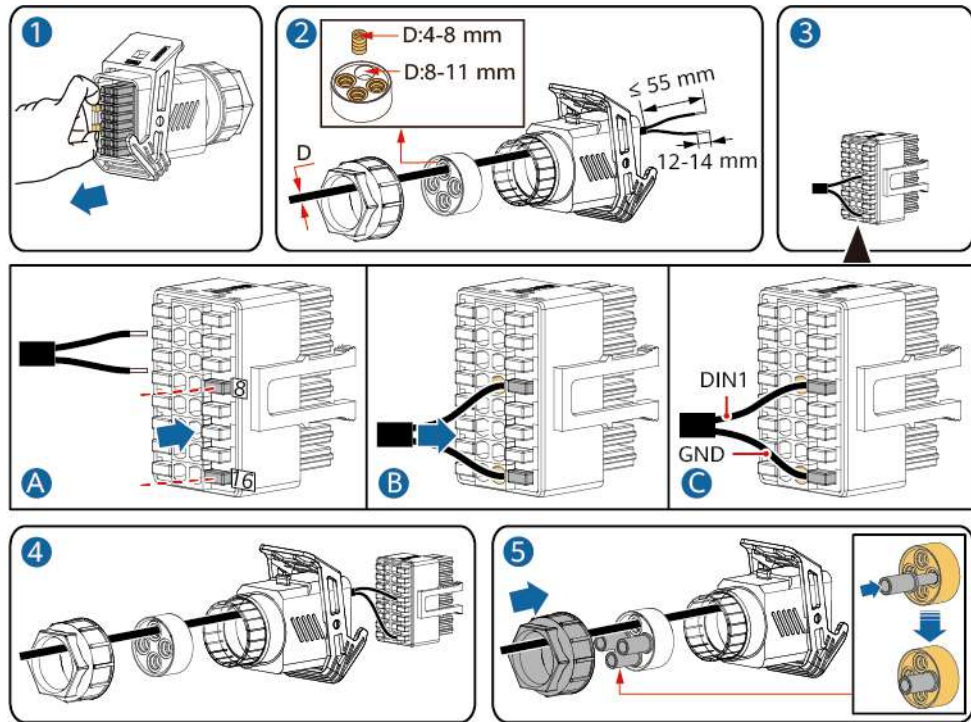
Figura 5-36 Instalación del cable
