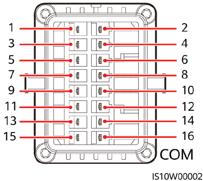
Figura 5-18 Definición de pines
